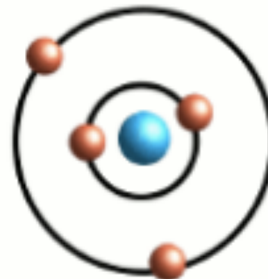
Beryllium
