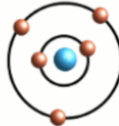
Bor
