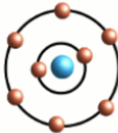
Sauerstoff
