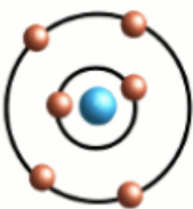
Kohlenstoff
