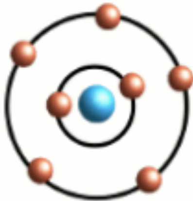
Stickstoff
